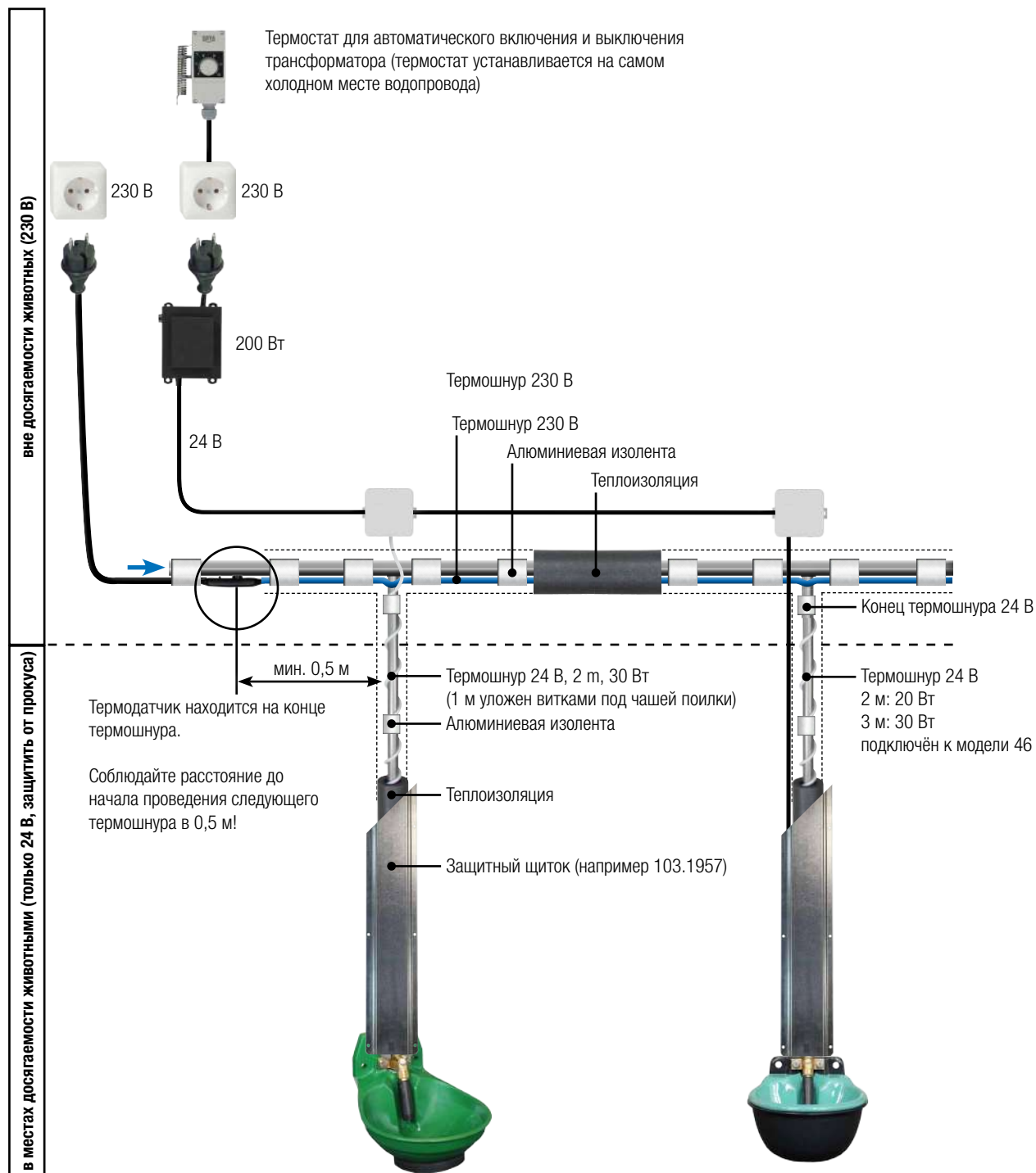
Модель 12P-НК (см. стр. 18) чаша с подогревом в комплекте с термошнуром: 24 В, 30 Вт = общая мощность: 30 Вт
